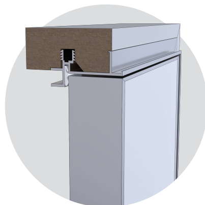
Полотно внешнего открывания
